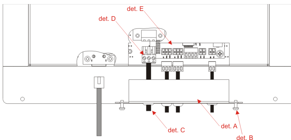
det. A – connectors cover; det. B – fixing screws; det. C – cable; det. D – plug; det. E – extender module;
